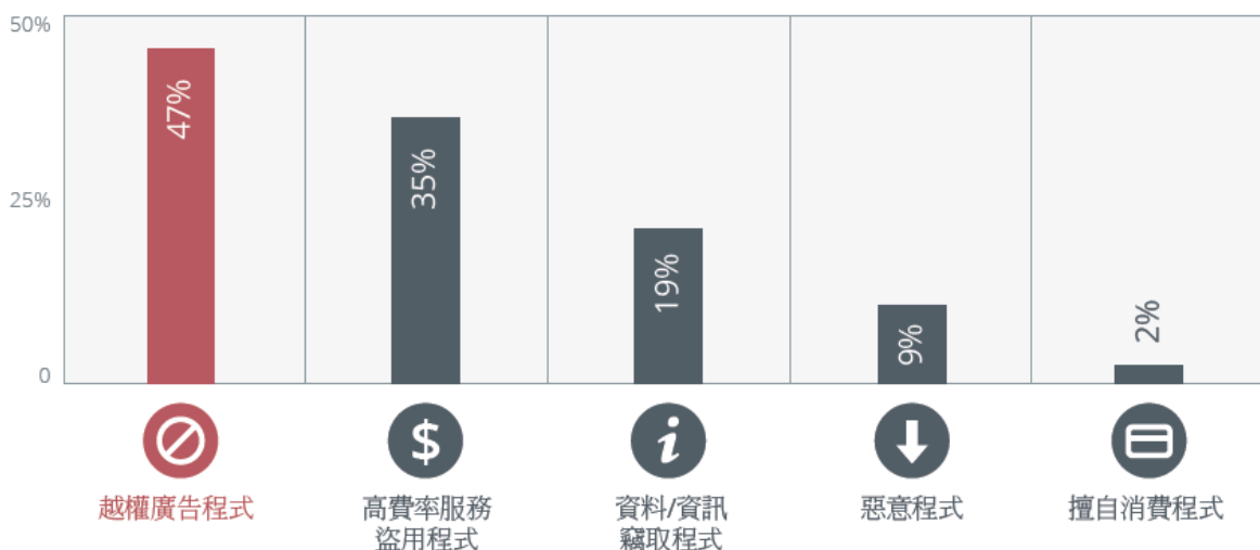
Android 領先威脅類型分布比例
